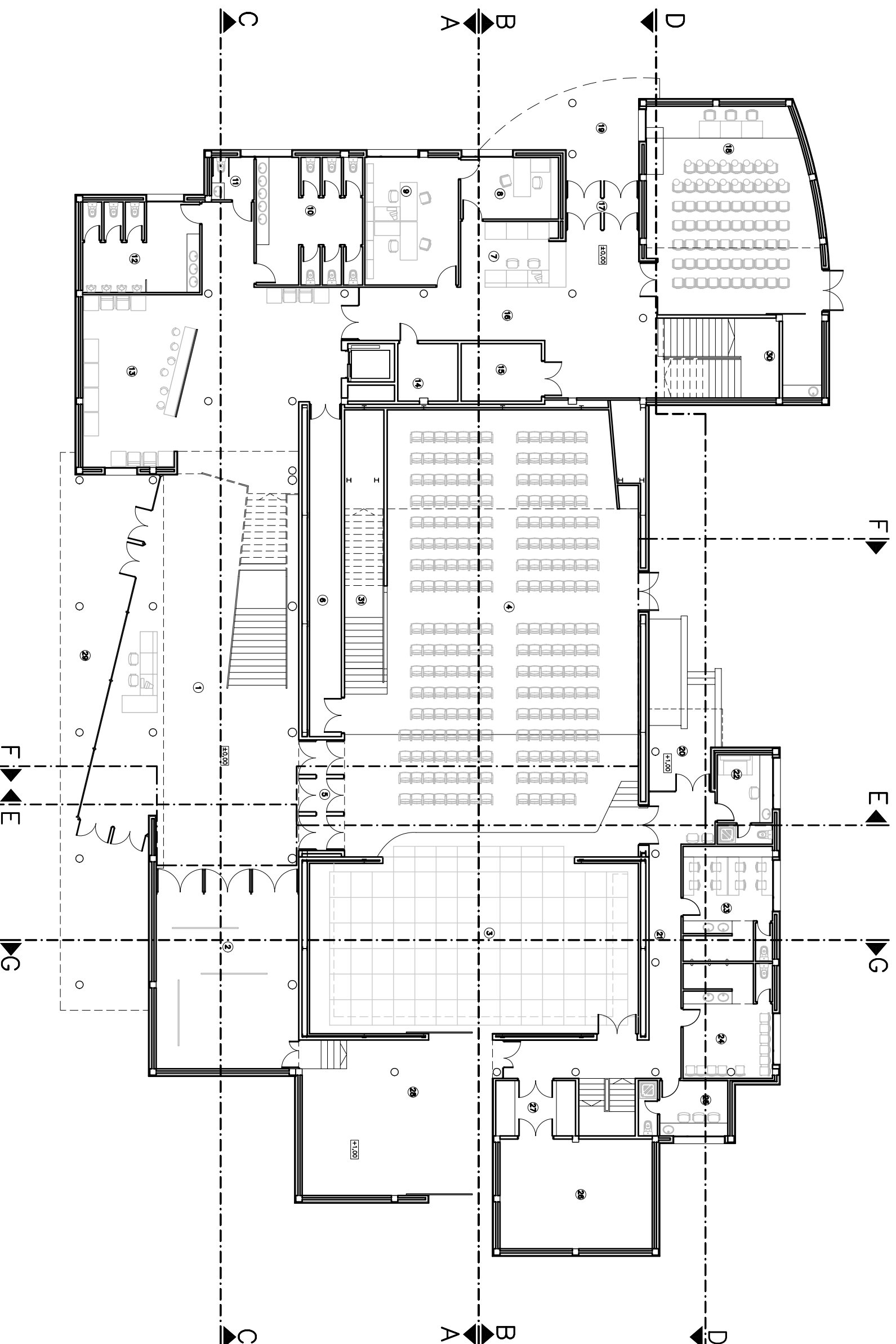
PLANTA BAIXA
